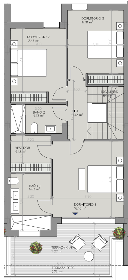
PLANTA PRIMERA
