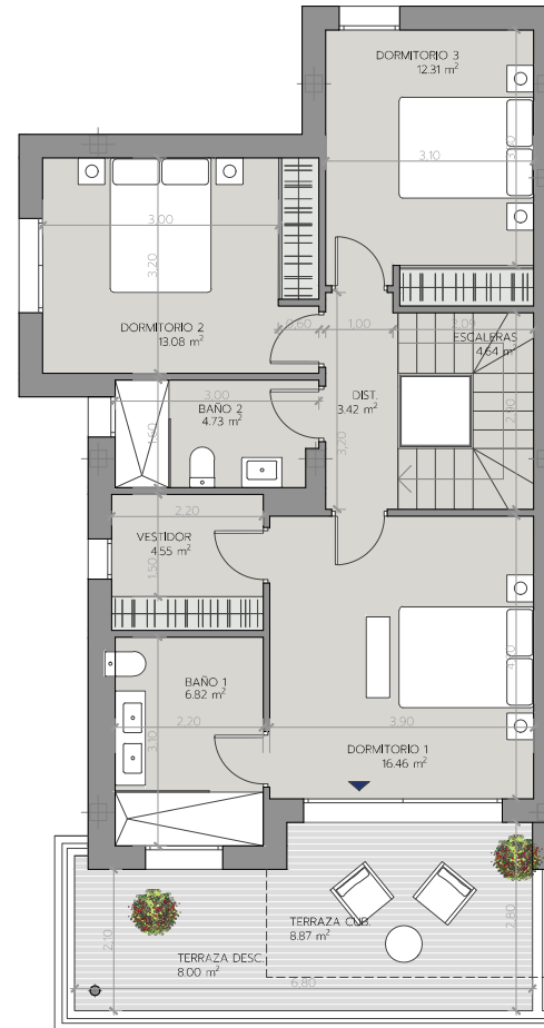
PLANTA PRIMERA
