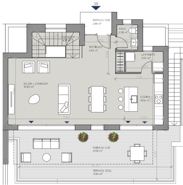
PLANTA PRIMERA
