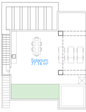
Solarium (E:1/200)
