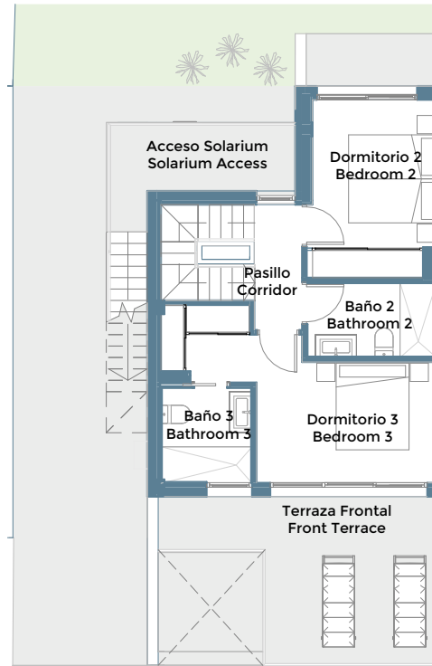
Planta Primera First Floor
