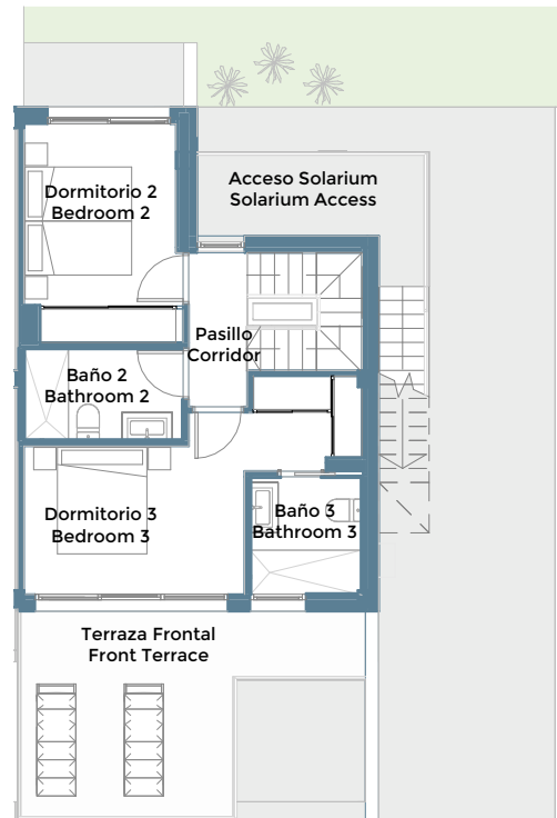
Planta Primera First Floor
