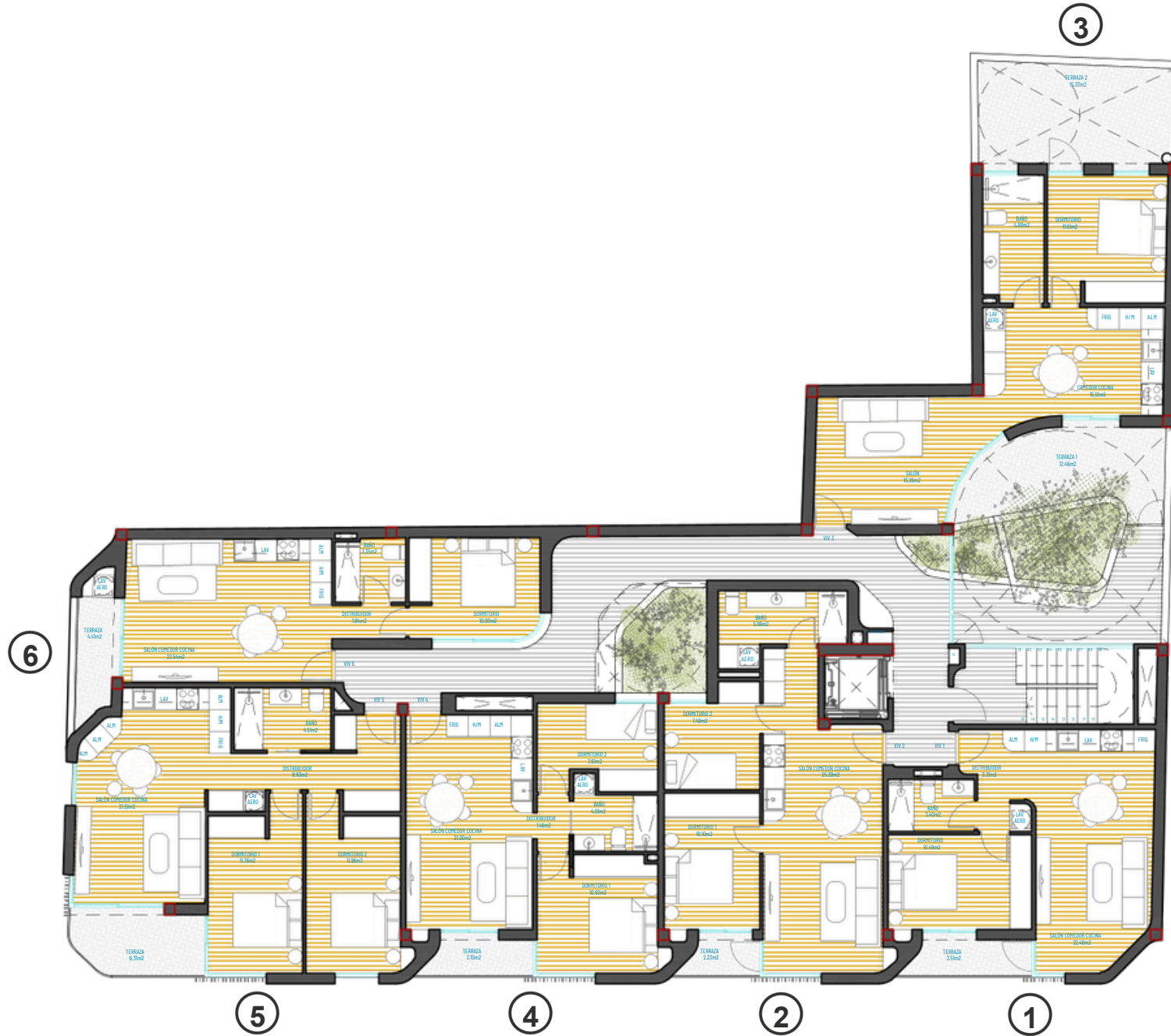
PLANTA PRIMERA
