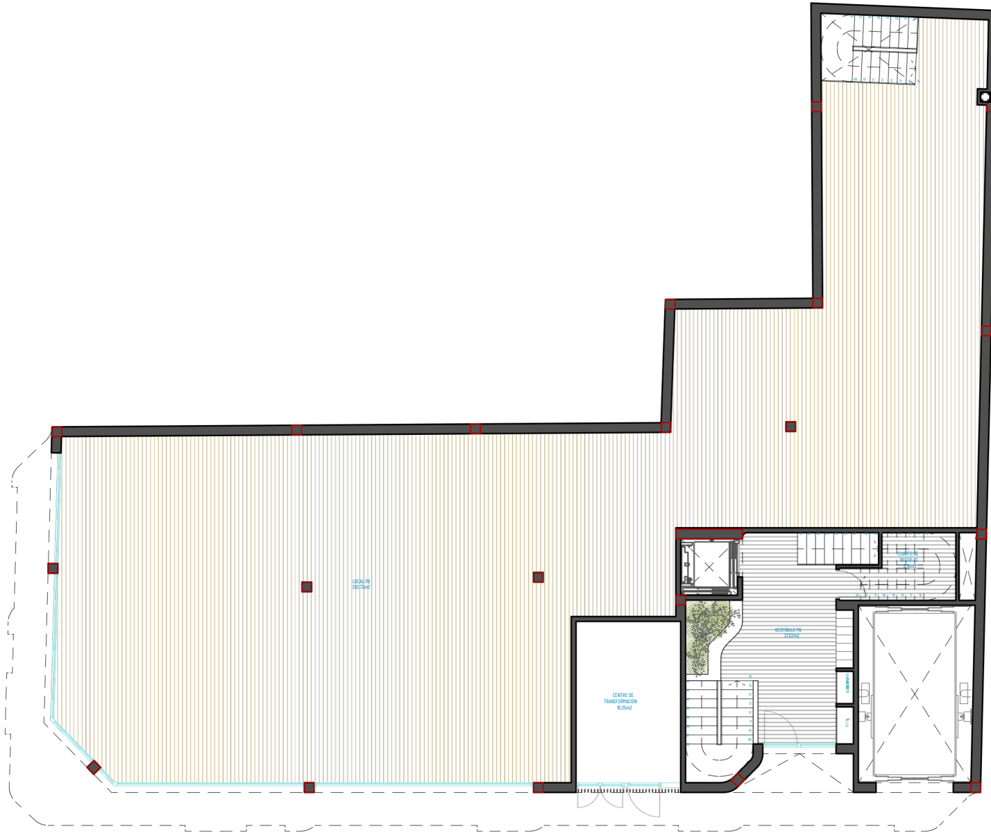
PLANTA BAJA
