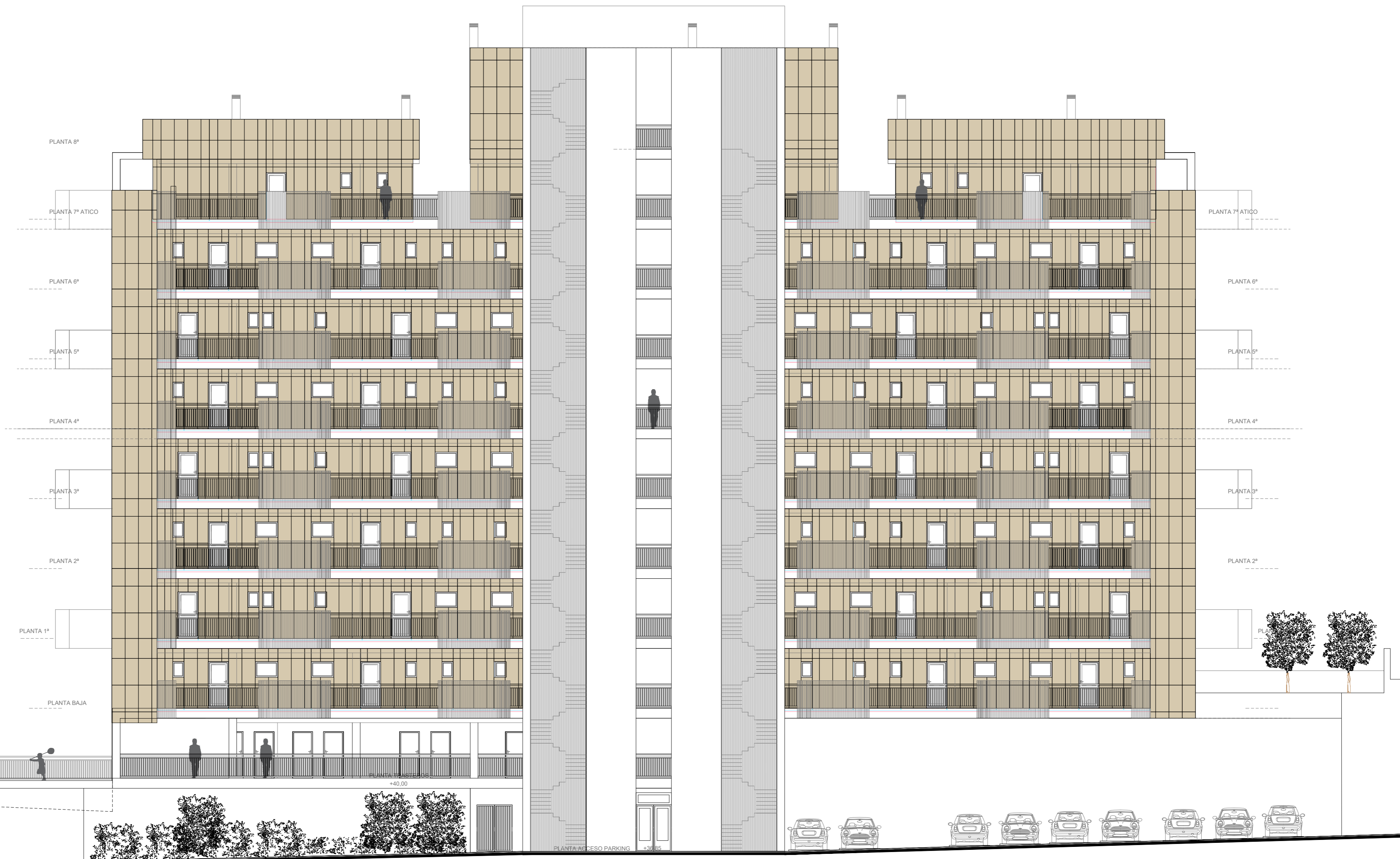
ALZADO POSTERIOR
