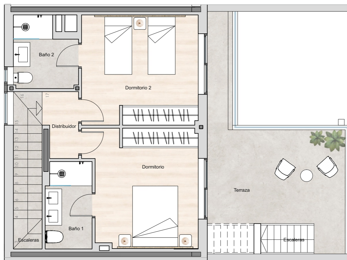
PLANTA PRIMERA
