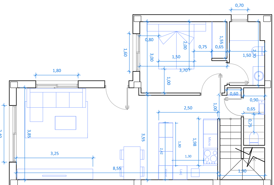
PLANTA BAJA
