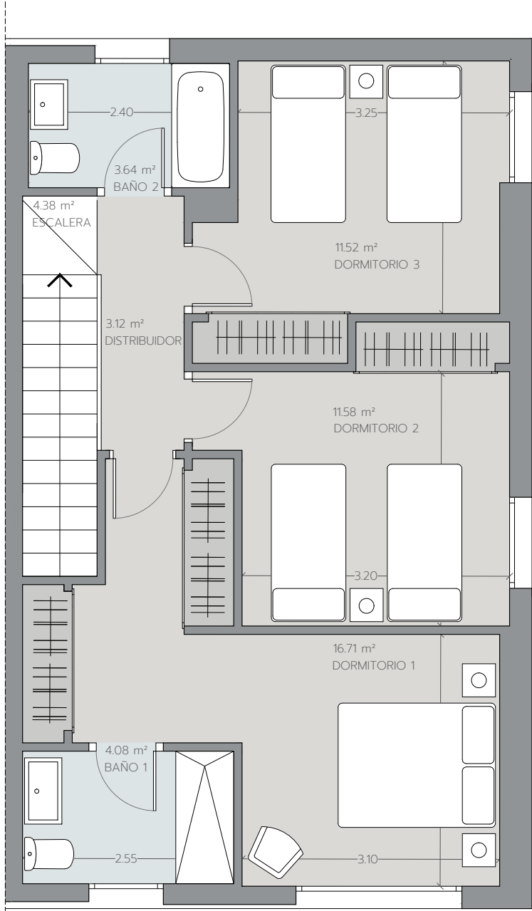
PLANTA PRIMERA
