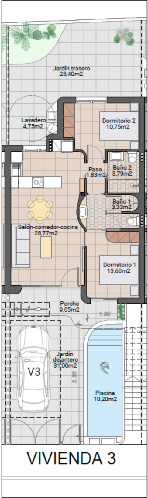
PLANTA BAJA
