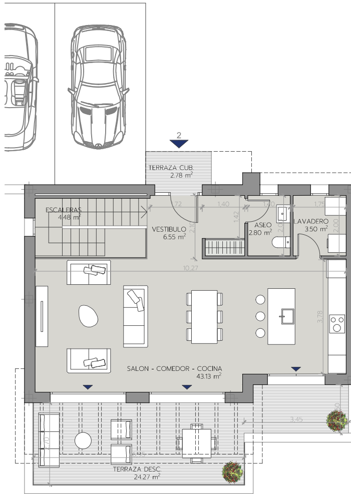
PLANTA PRIMERA
