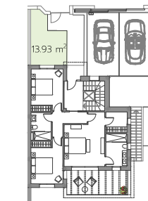
PLANTA ACCESO
