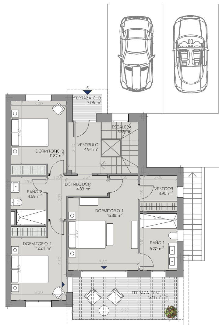
PLANTA PRIMERA
