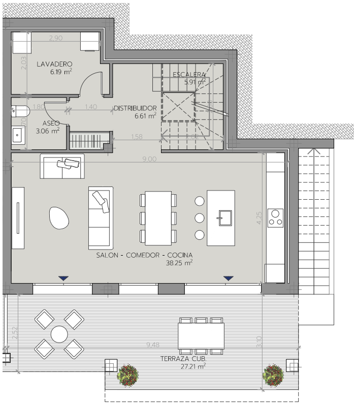
PLANTA BAJA
