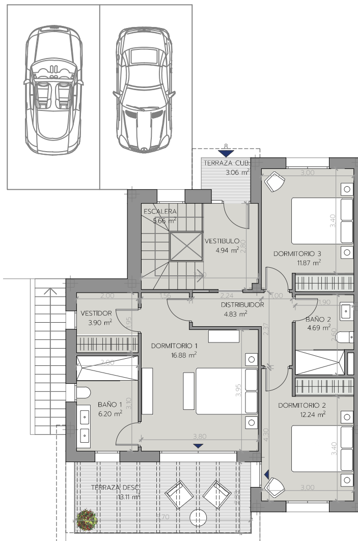
PLANTA PRIMERA
