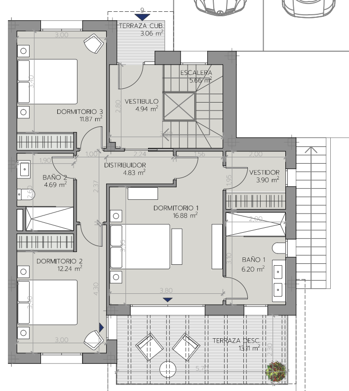
PLANTA PRIMERA
