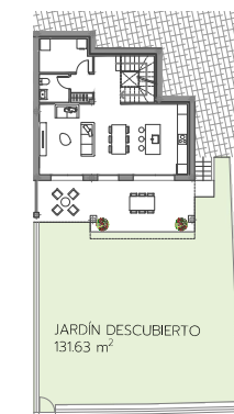
PLANTA DE JARDÍN
