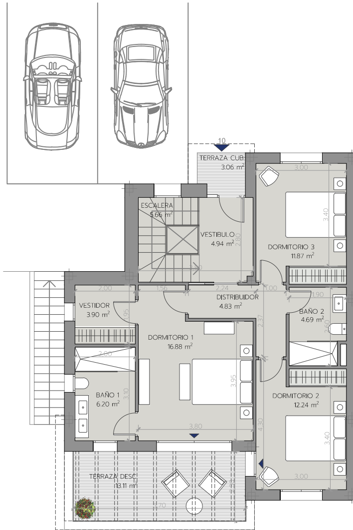
PLANTA PRIMERA
