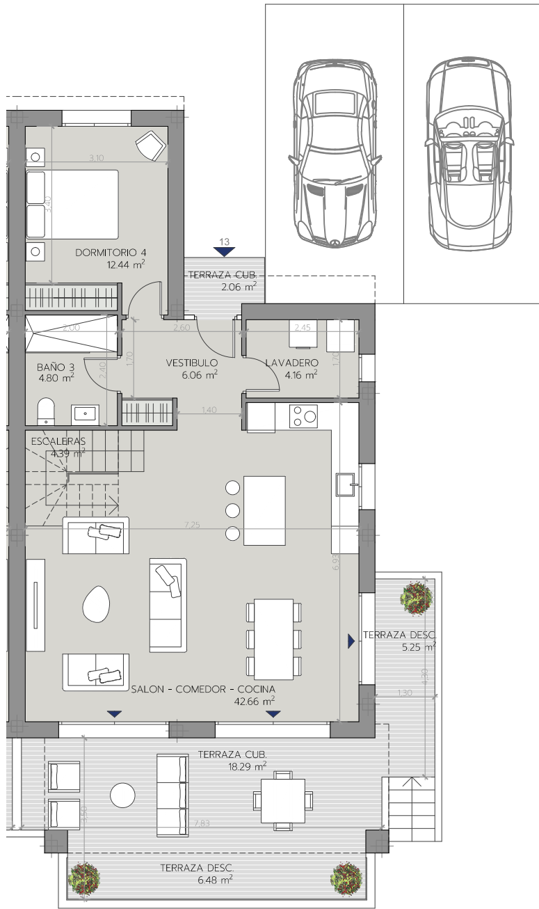
PLANTA BAJA
