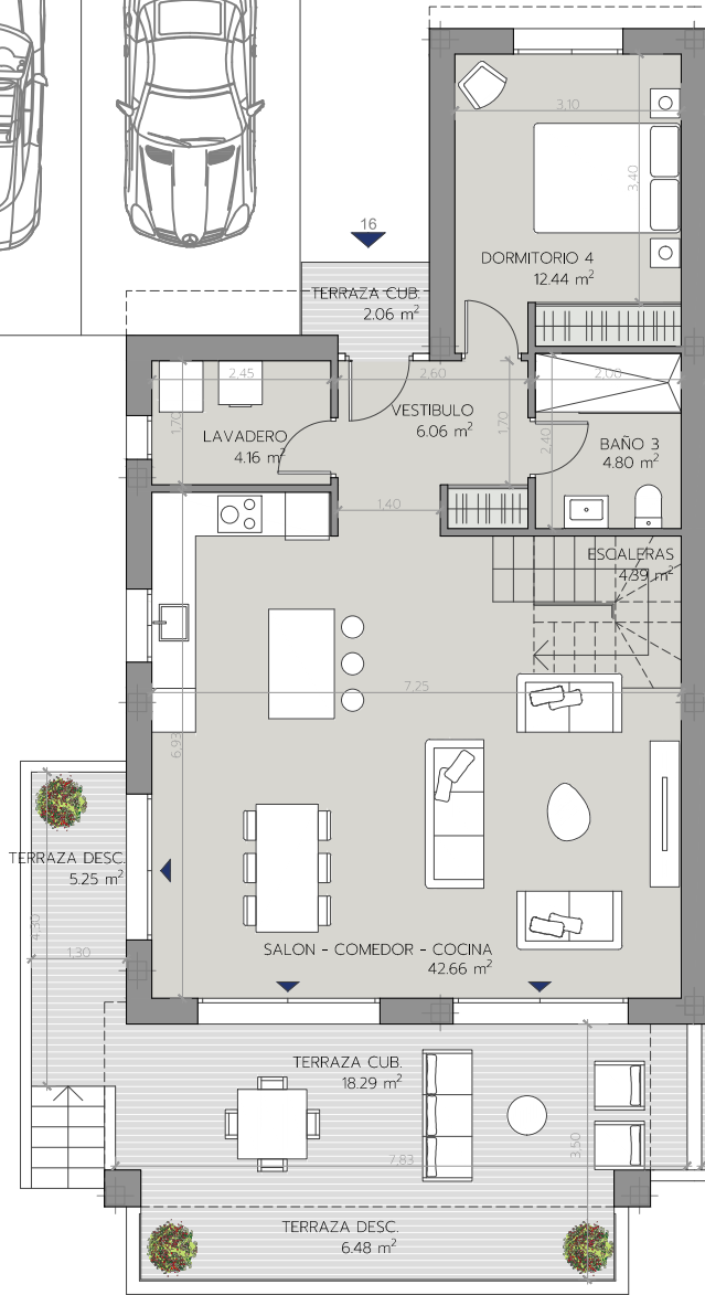
PLANTA BAJA
