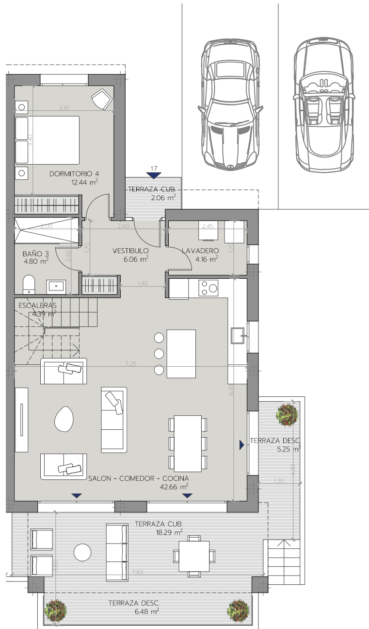
PLANTA BAJA
