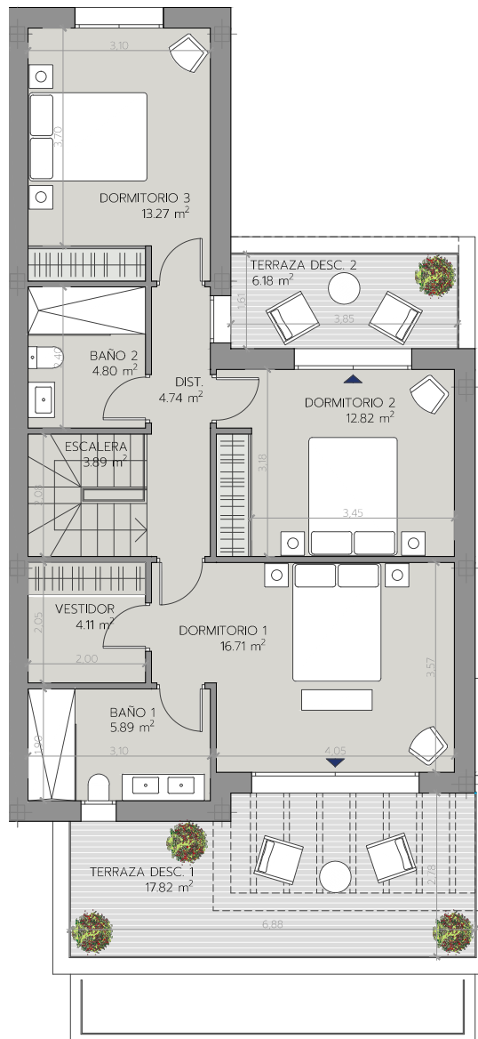
PLANTA PRIMERA
