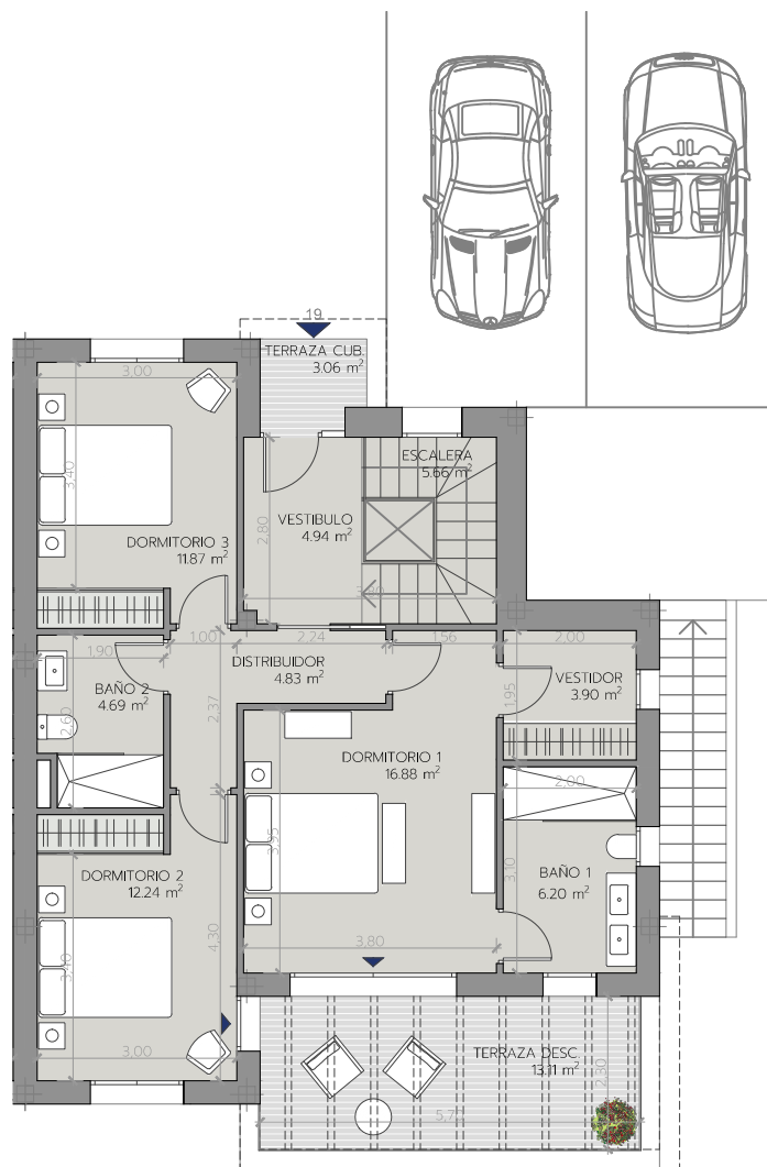
PLANTA PRIMERA
