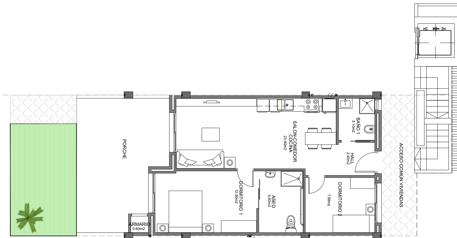
Planta Baja
