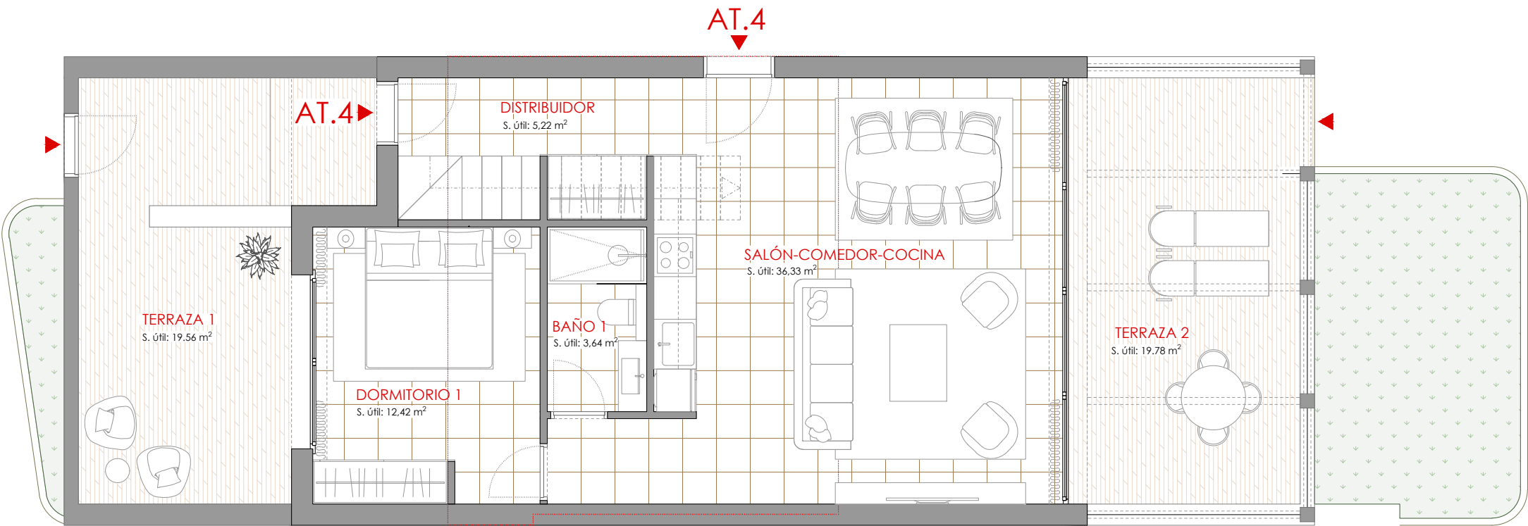
Planta baja
