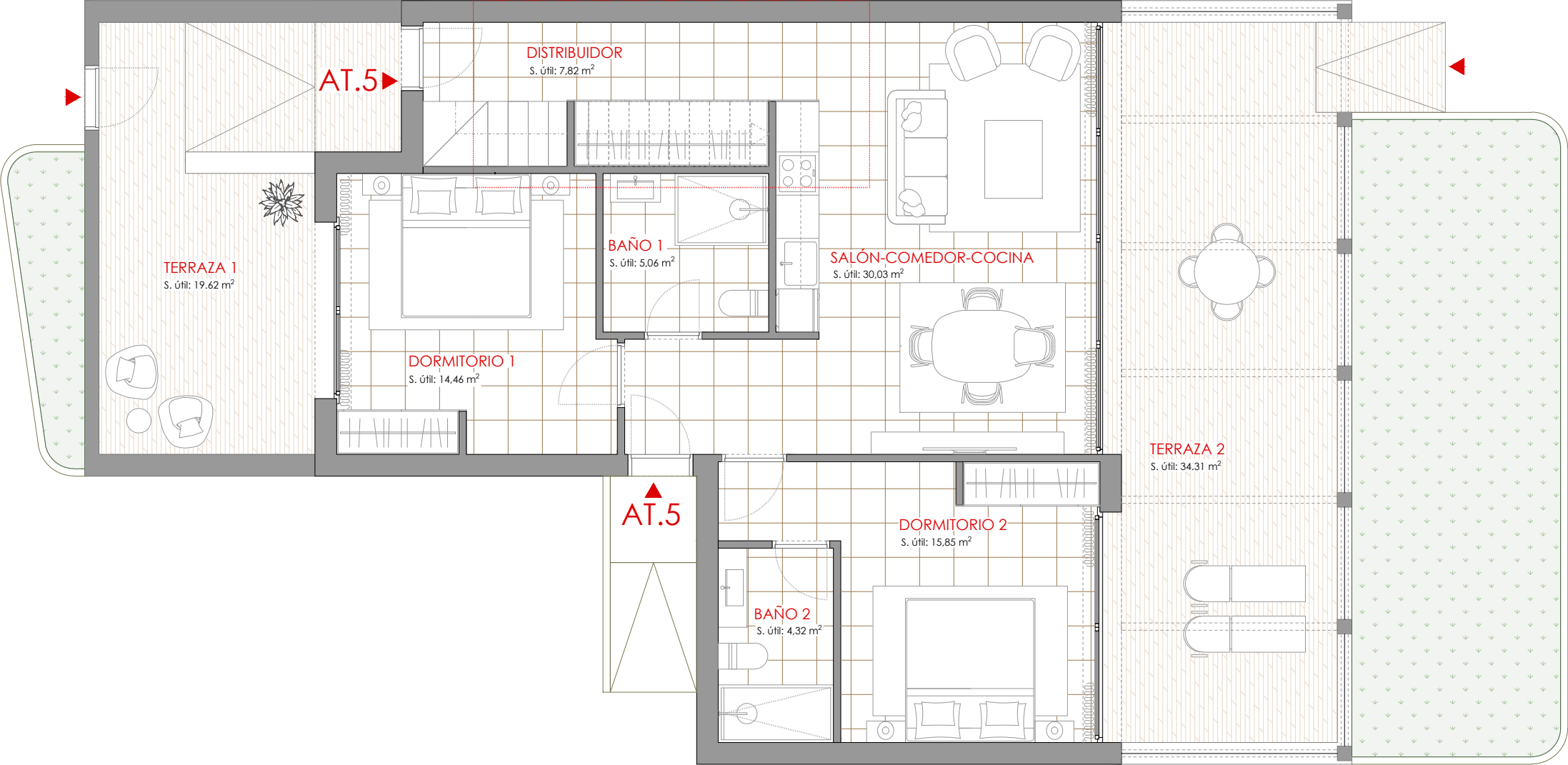
Planta baja
