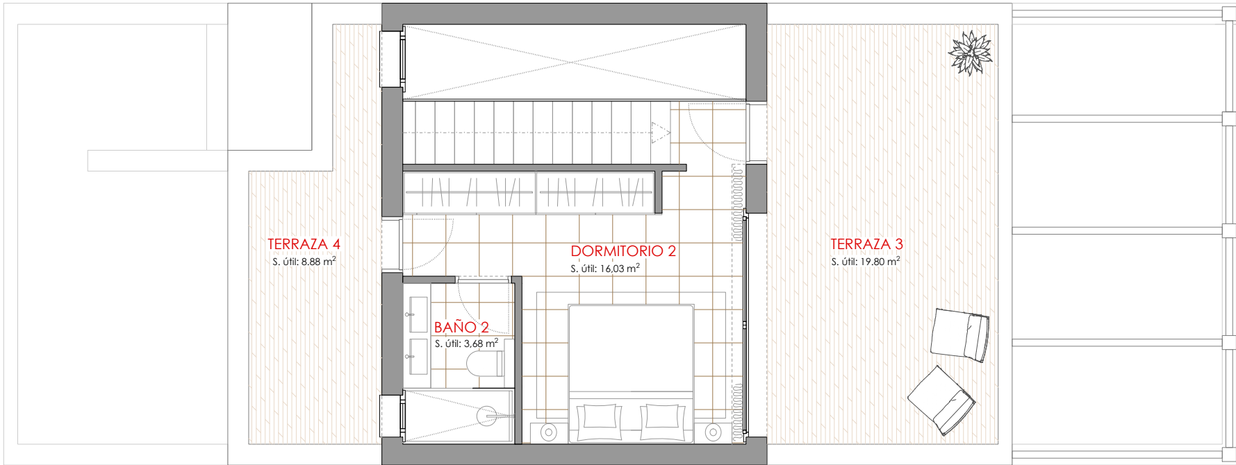
Planta primera
