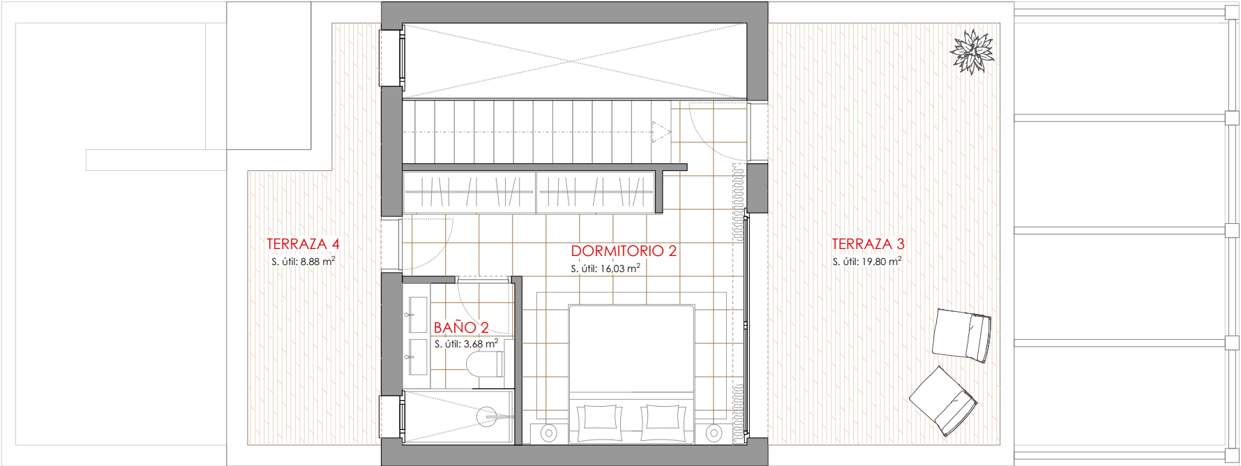
Planta primera
