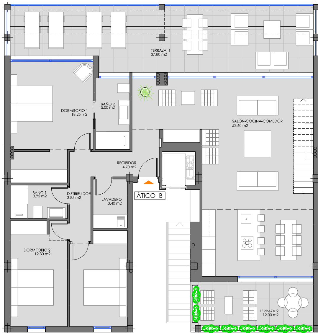
PLANTA ÁTICO
