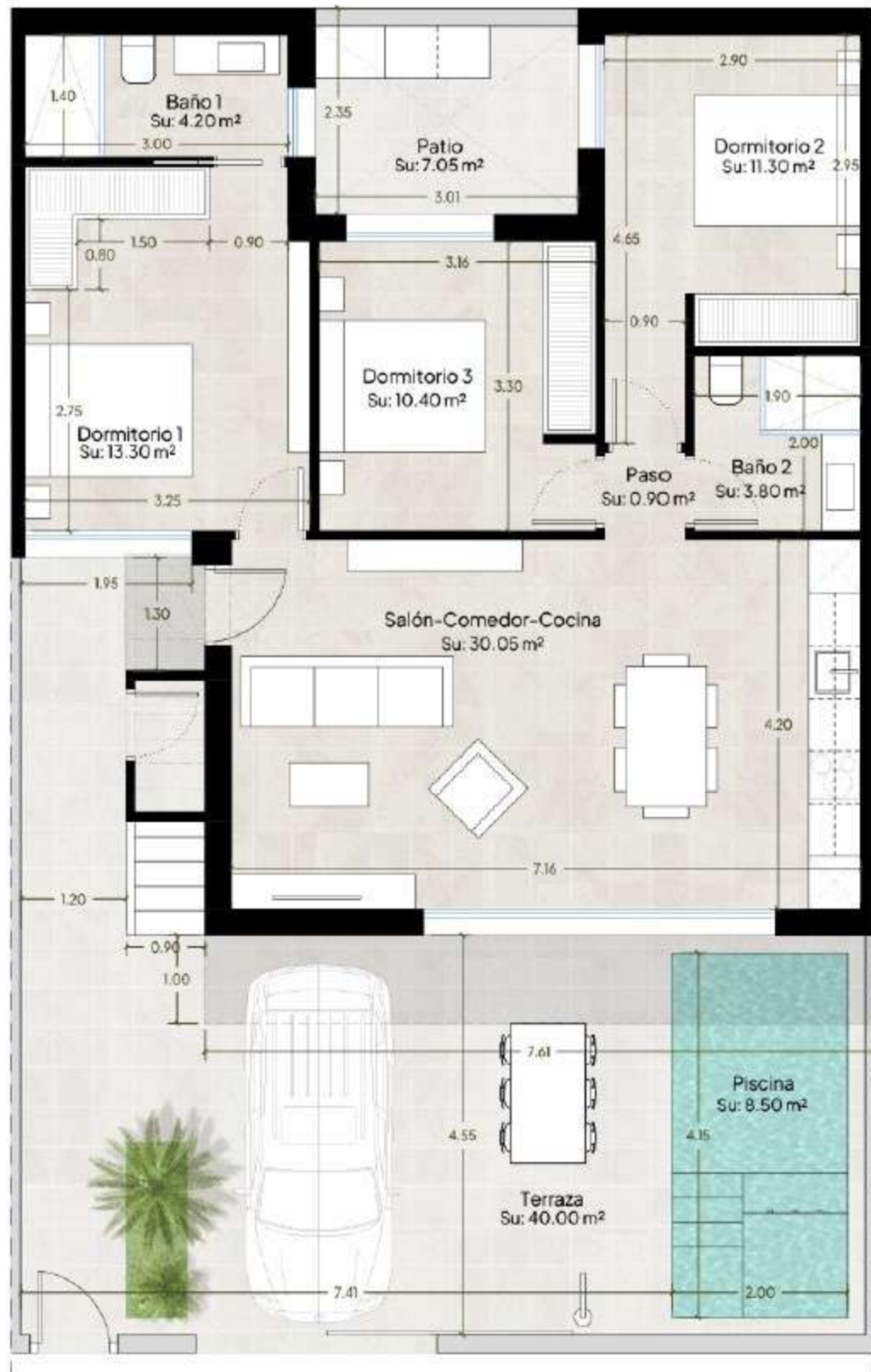
Planta Baja
