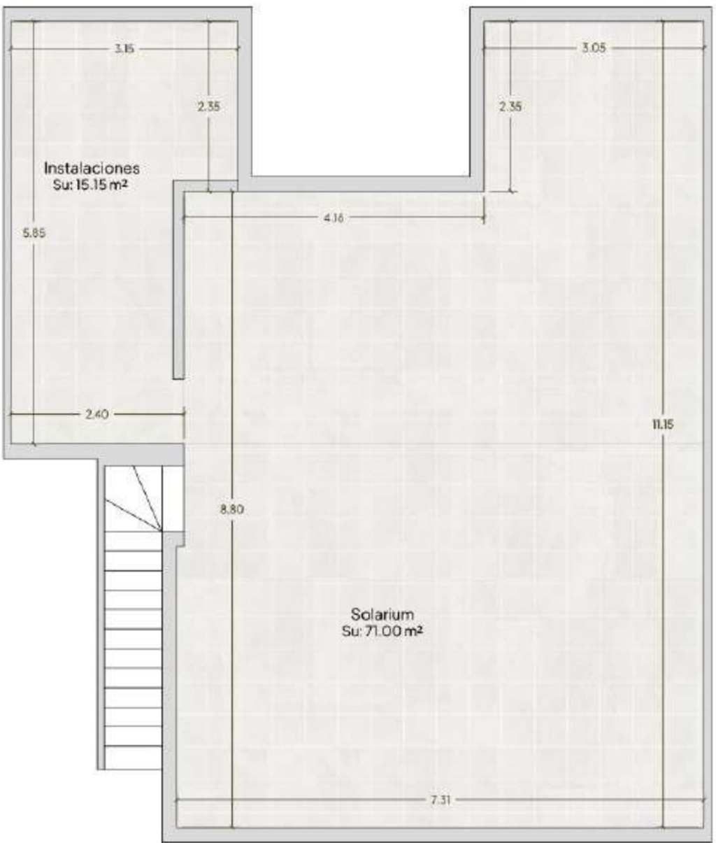
Solarium
