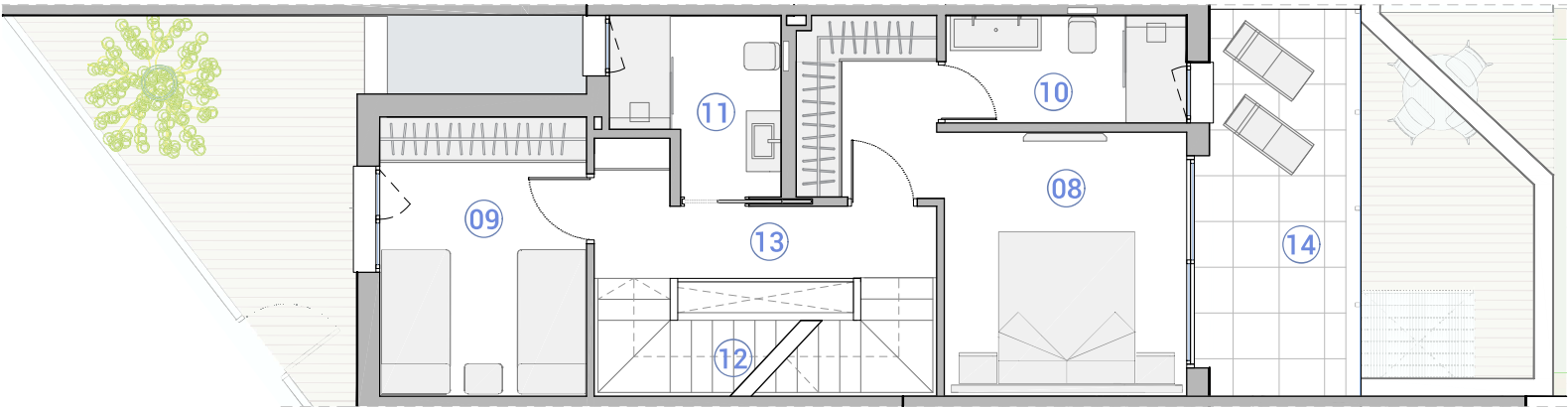
Planta / Floor Primera / First
