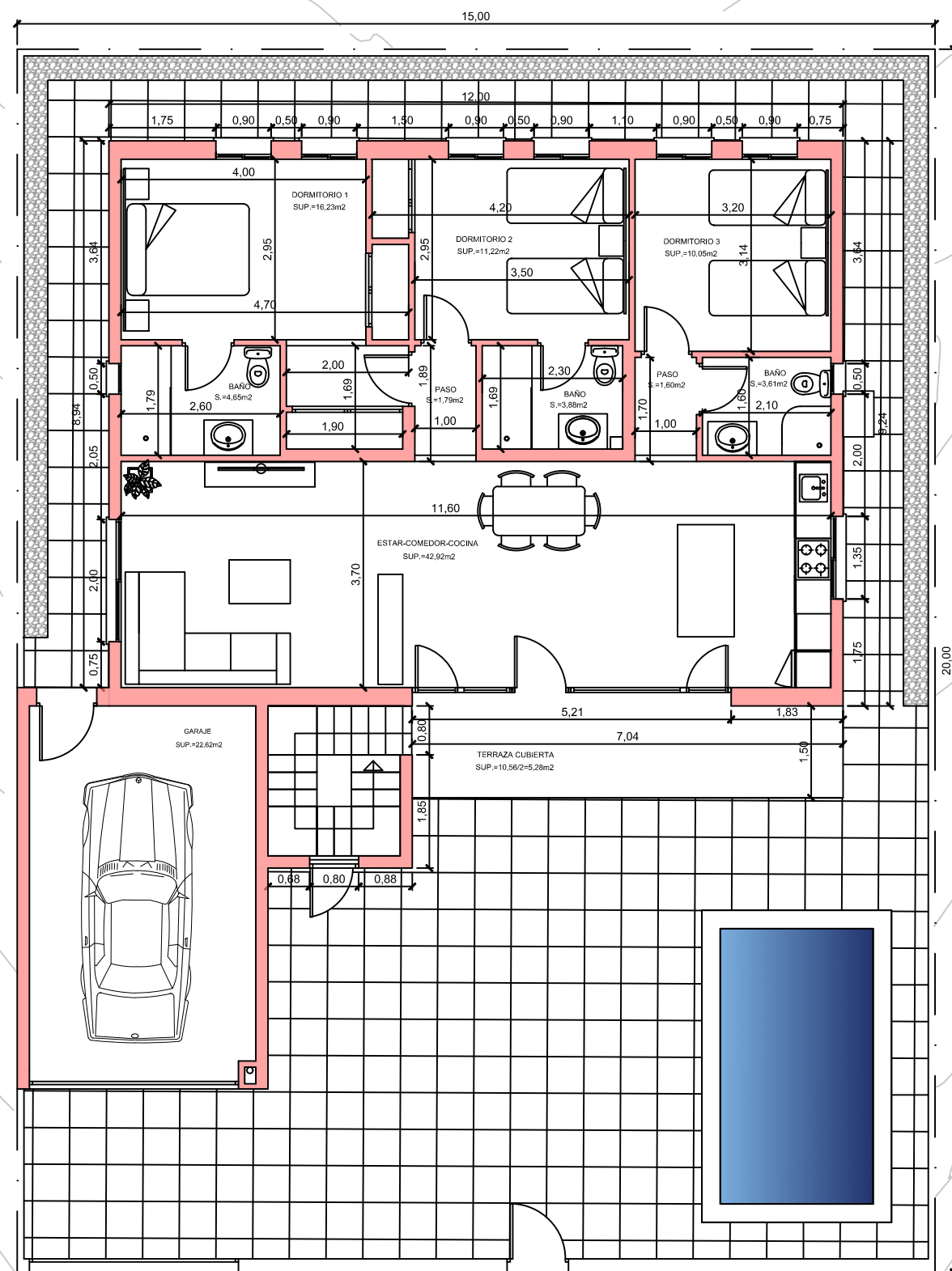
PLANTA BAJA
