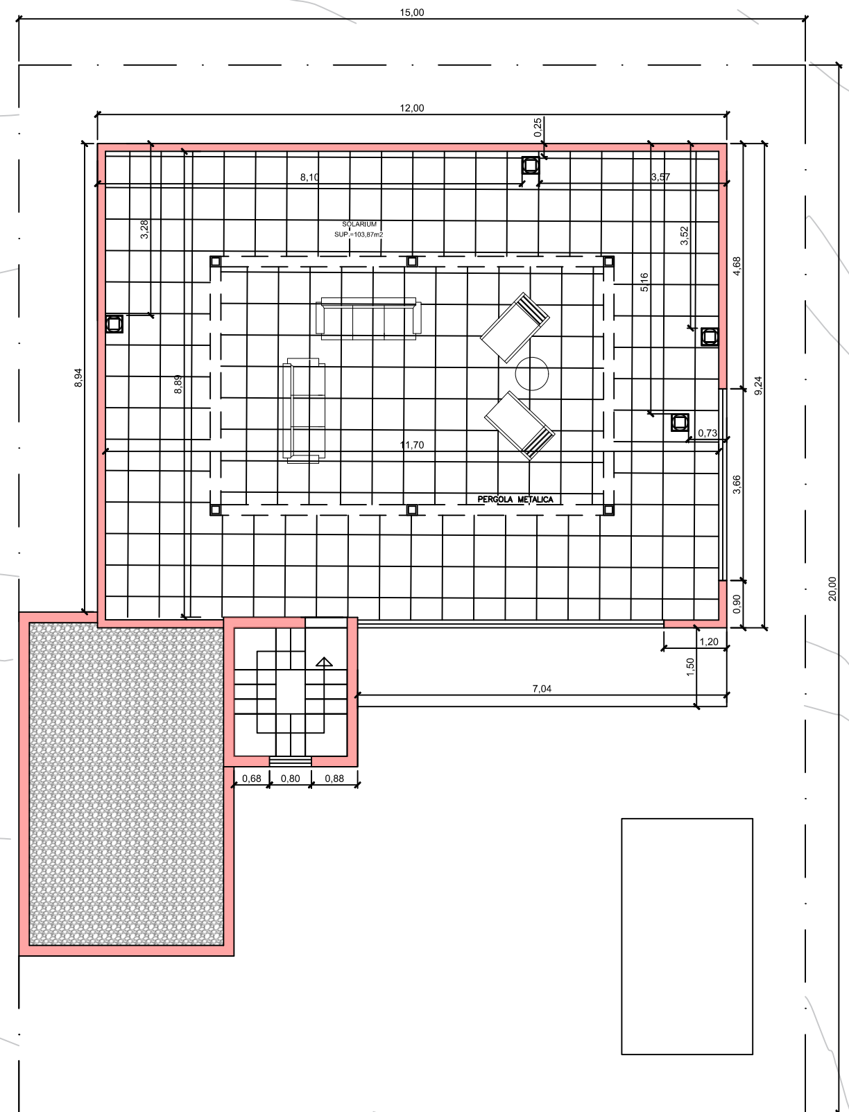
PLANTA SOLARIUM
