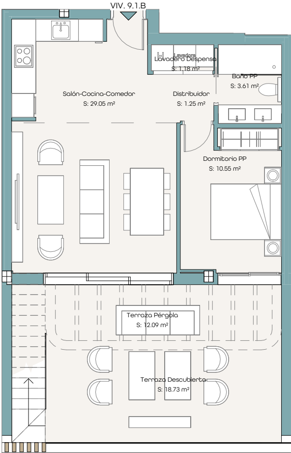
PLANTA PRIMERA
