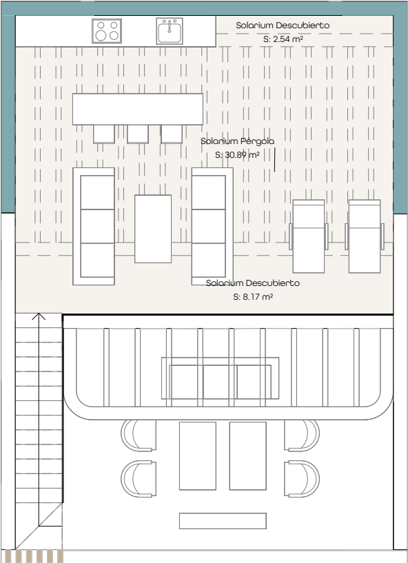
PLANTA SOLARIUM
