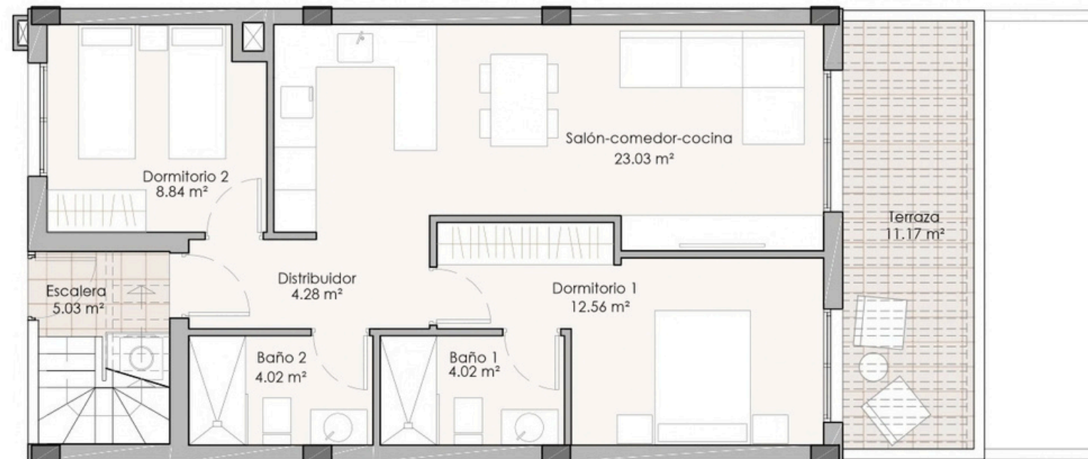
Planta Primera
