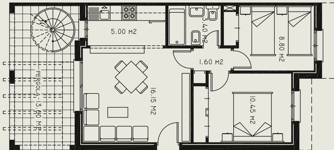
PLANTA BAJA
