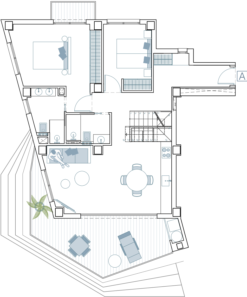
PLANTA QUINTA
