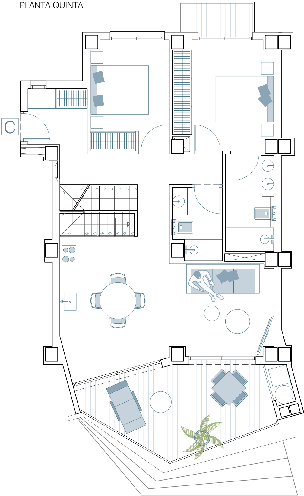
PLANTA QUINTA
